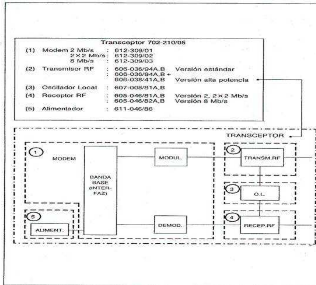
Fig. 6 - Composición del transceptor
