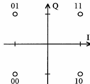
Constelación 4PSK
