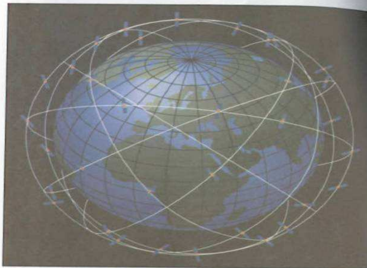
Lámina 32 La constelación Globalstar consiste de 48 satélites en órbita baja. (Cortesía de Globalstar). Véase también la Fig. 8-20, pp 453.
