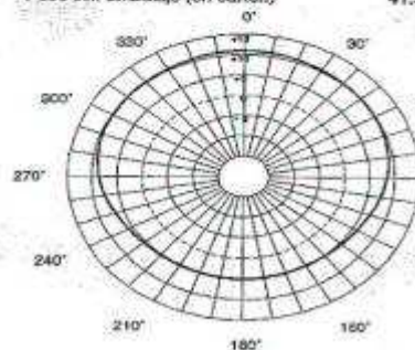
Diagrama unidireccional
