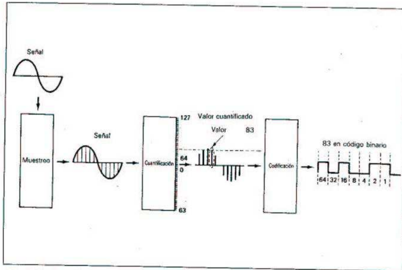
Fig. 5.2. La técnica de modulación MIC se basa en el muestreo, cuantificación y codificación de una señal analógica, para su transformación en digital.
