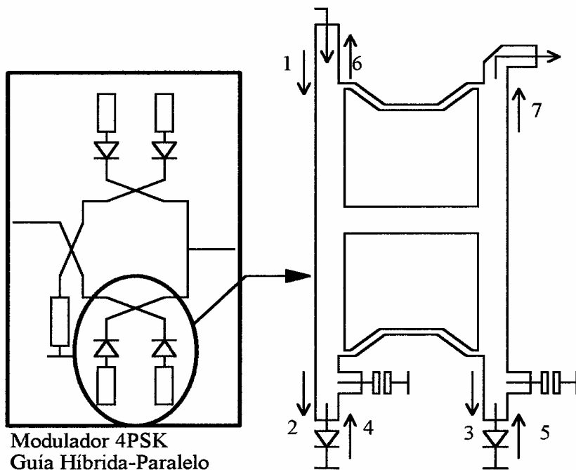
Modulador 4PSK
