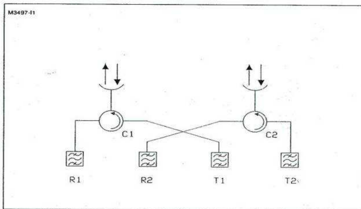
Fig. 10 - Sistema 1 + 1 heterofrecuencia con dos antenas
