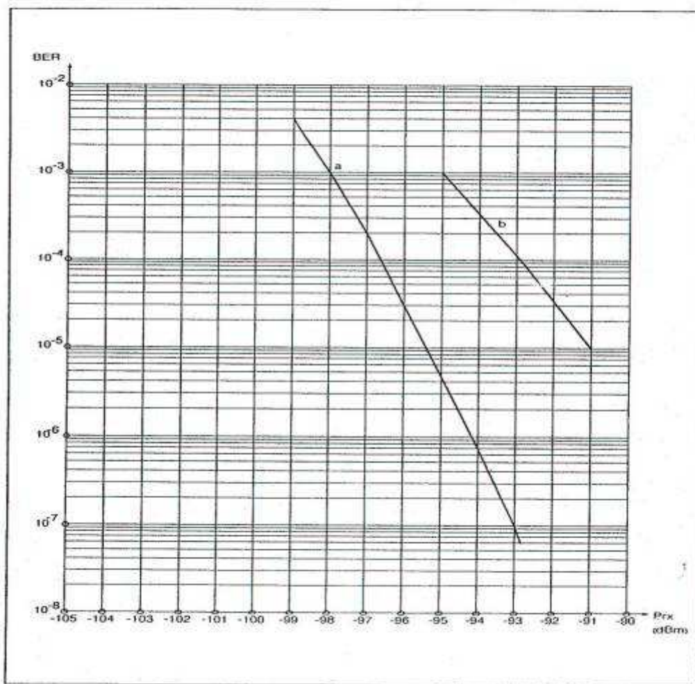
Fig. 13 - Curva de BER a 2 Mb/s
