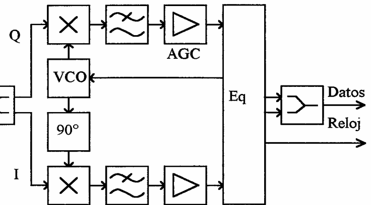
Demodulador 4PSK
