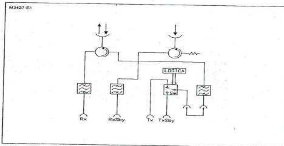
Fig. 8 - Sistema 1 + 1 Hot Stand-by - Dos antenas
