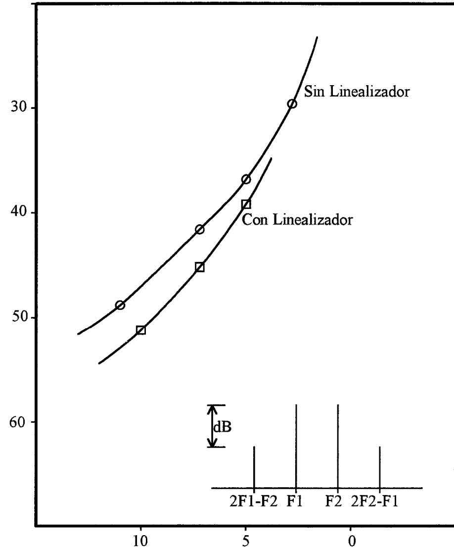
Intermodulación dB vs Backoff dB
