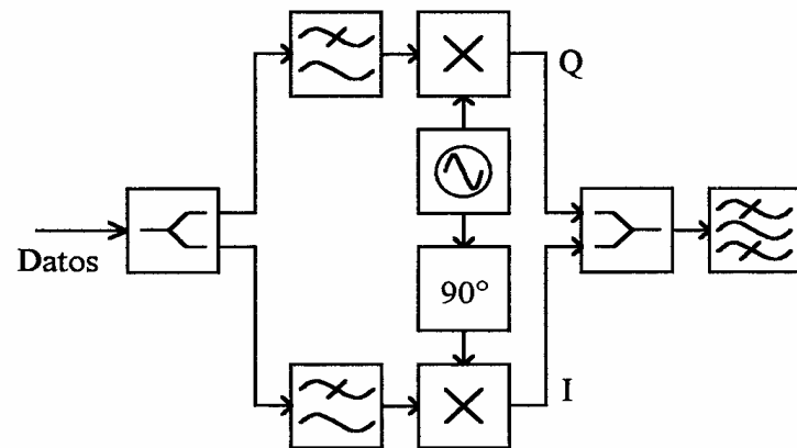
Modulador 4PSK
