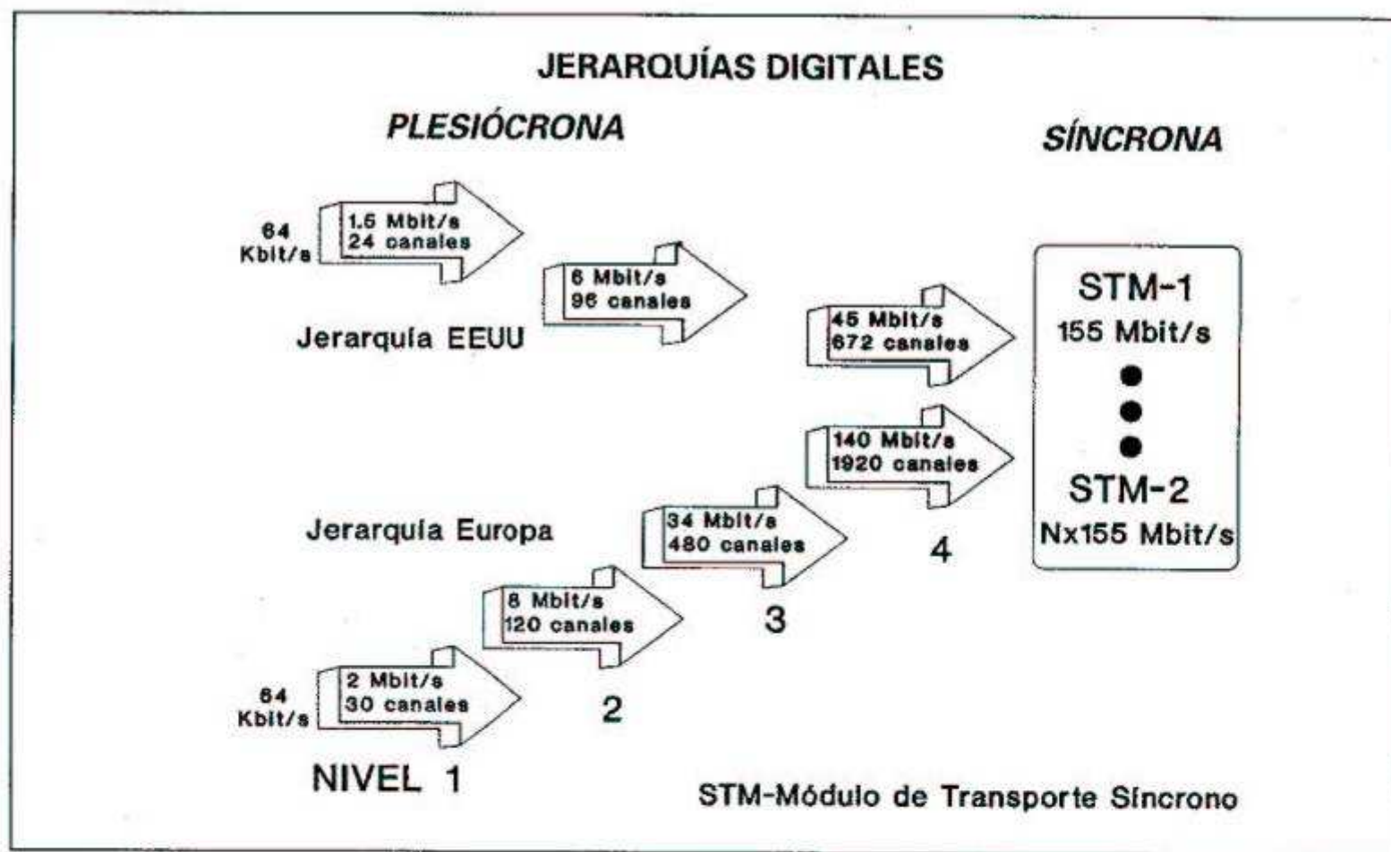
Fig. 5.5. Evolución de la jerarquía digital plesiócrons (JDP) hacia la síncrona (JDS).
