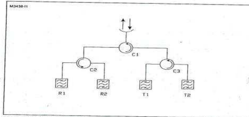
Fig. 9 - Sistema 1 + 1 heterofrecuencia
