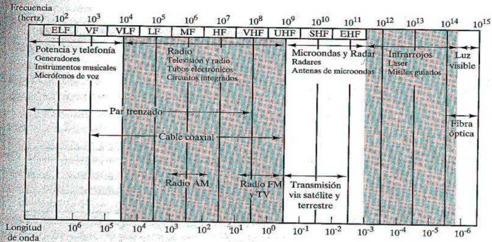
FIGURA 3.1 Espectro electromagnético para las telecomunicaciones.
