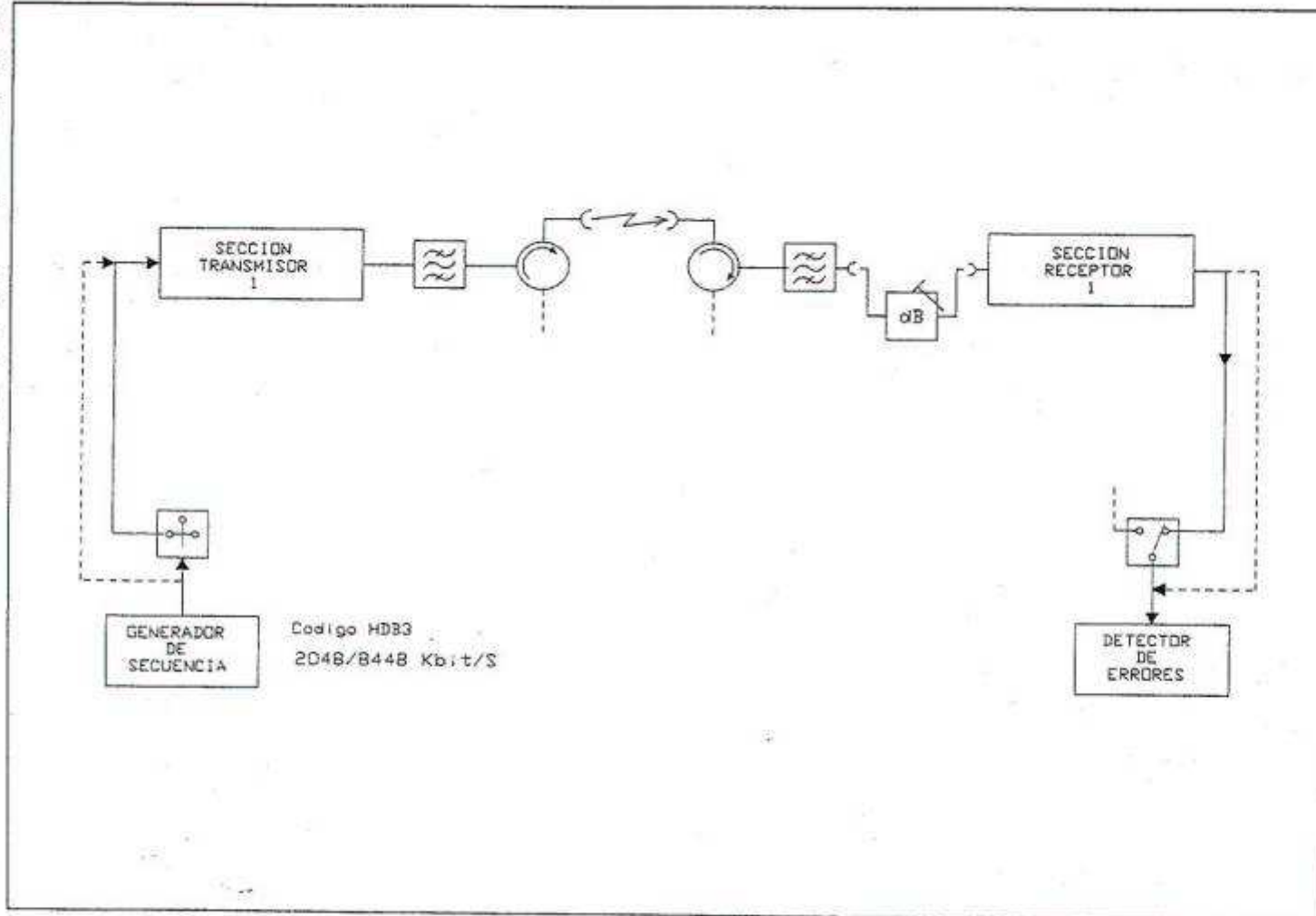
Fig. 10 - Esquema de medición de la BER en el flujo a 2/8 Mb/s
