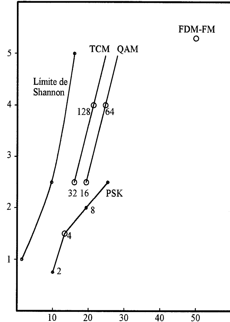
Eficiencia Espectral (bit/seg/Hz) vs C/N dB
