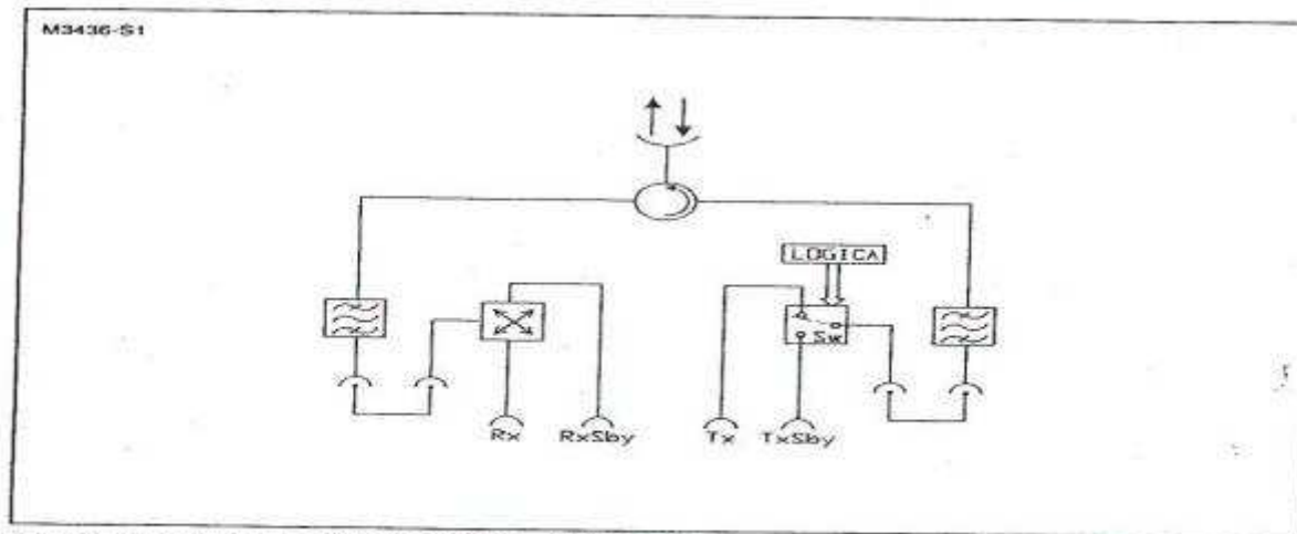
Fig. 7 - Sistema 1 + 1 Hot Stand-by - Antena única
