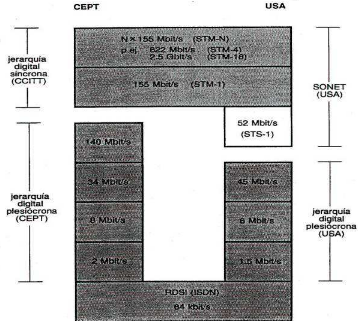
Fig. 4 Comparación de las jerarquías múltiplex CEPT y USA
